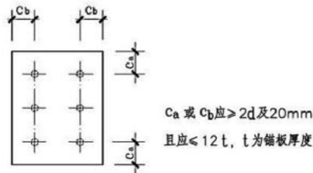
图D.3.1 锚筋到锚板的边距
