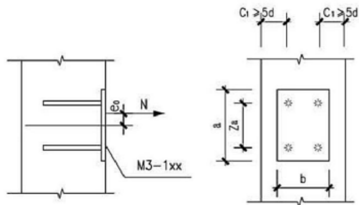
拉弯预埋件
