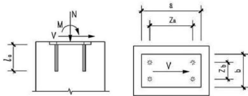
无抗剪钢板的压弯剪预埋件
