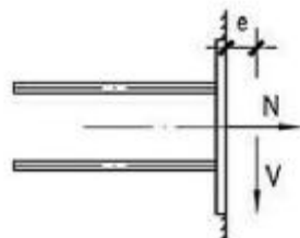
拉弯剪预埋件
