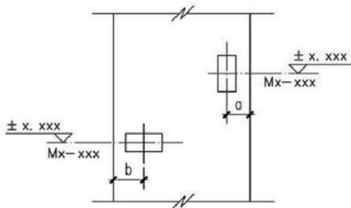
图A.3.1 预埋件在构件上的位置示意图
