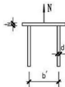
图 G. 2. 1 直锚筋轴心受拉预埋件
