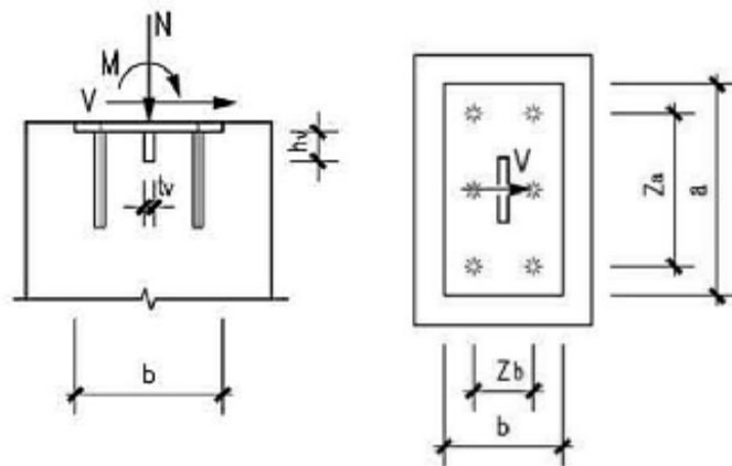
有抗剪钢板的压弯剪预埋件
