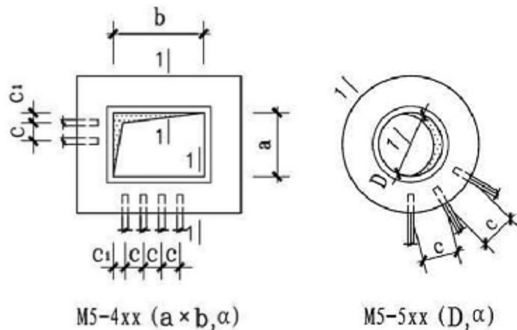
护边框预埋件
