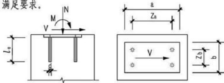
无抗剪钢板的压弯剪预埋件
