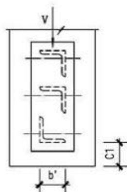
图 G.3.4 角钢锚筋的受剪预埋件
