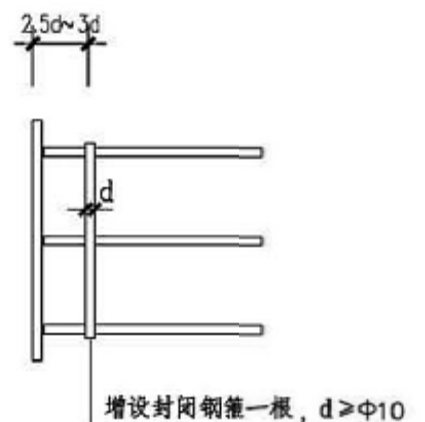
图A. 3.5 地震区受力锚筋构造要求
