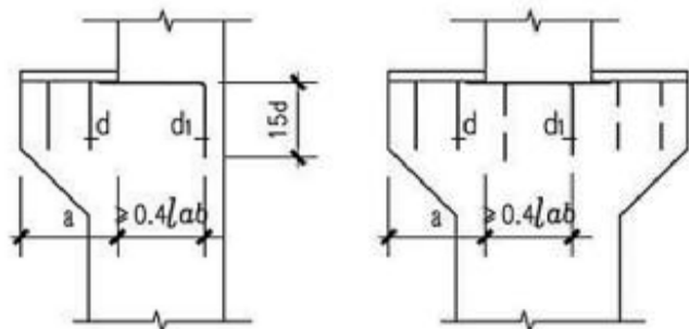
拉筋现场弯折示意图
