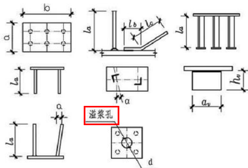
图8.3 预埋件加工
