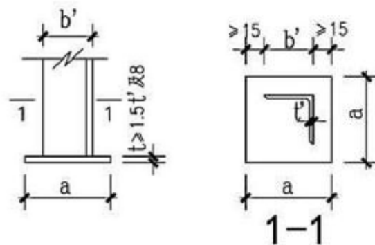
图D.4.2 角钢锚筋端锚板的尺寸
