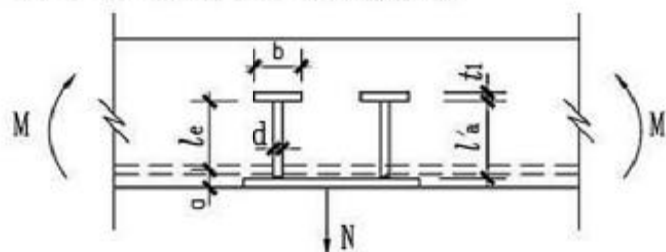
图E.1.1 锚筋端部加焊锚板
