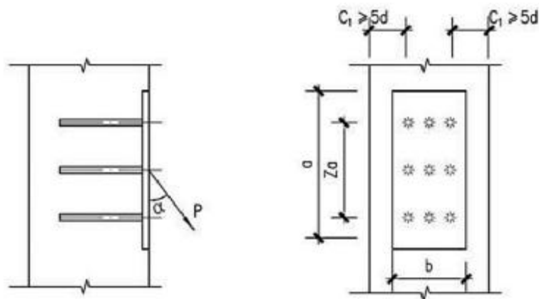
拉剪预埋件
