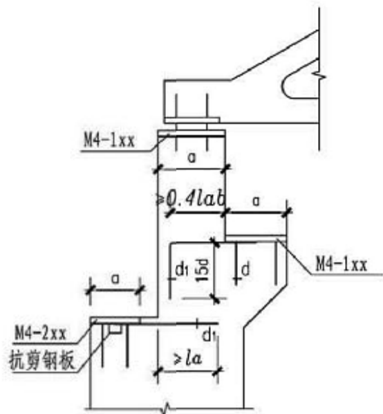
压弯剪预埋件应用部位举例
