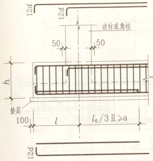
端部等截面外伸构造
