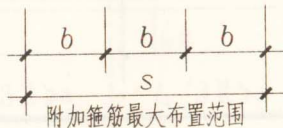
附加箍筋最大布置范围
