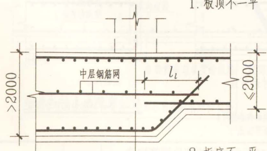
3. 板底不一平
