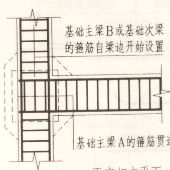
丁字相交平面(一)
