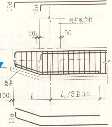
端部变截面外伸构造(二) (基础梁顶与基础板顶一平)
