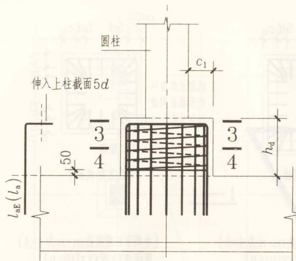
圆柱状上柱墩 SZD
