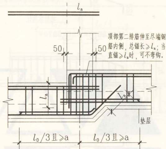
底部第二排筋伸至末端钢筋内侧, 总锚长 \geq l_a ; 当直锚 \geq l_a 时, 可不弯钩。
