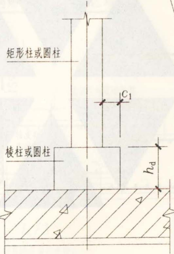
基础平板上柱墩SZD (柱墩为棱柱或圆柱形状)
