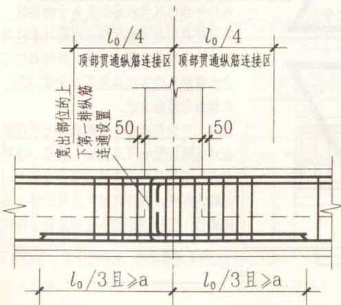
柱两边梁宽不同钢筋构造
