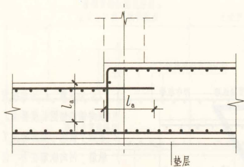
1. 板顶有高差
