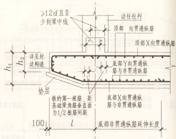
端部变截面外伸构造(二)(基础板顶一平)
