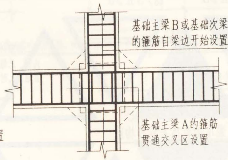
十字相交平面
