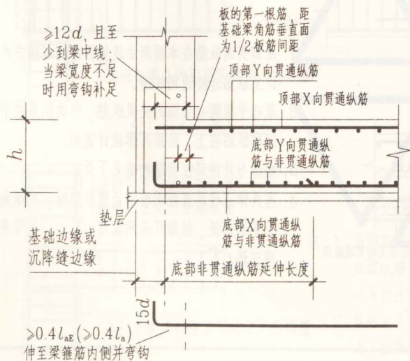
端部无外伸构造(跨中底部无Y向非贯通纵筋)
