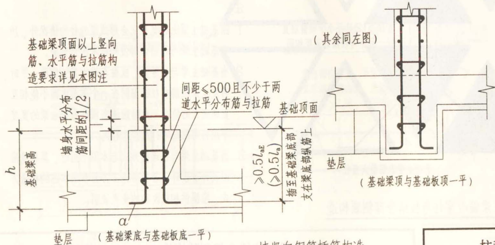
墙竖向钢筋插筋构造
