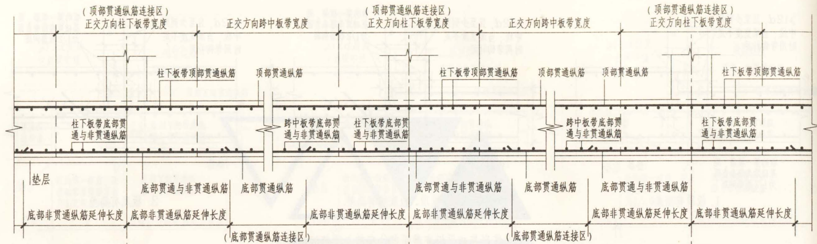
柱下板带 ZXB 纵向钢筋构造
