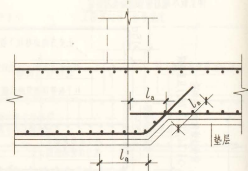
3. 板底有高差
