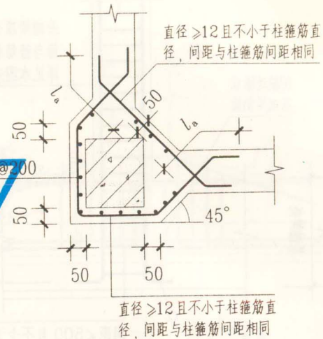
无外伸基础主梁与角柱结合部侧腋构造
