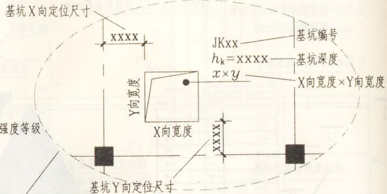
基坑JK直接引注
