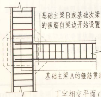
丁字相交平面(一)
