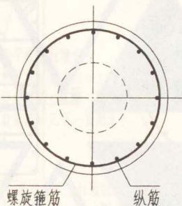
4—4
