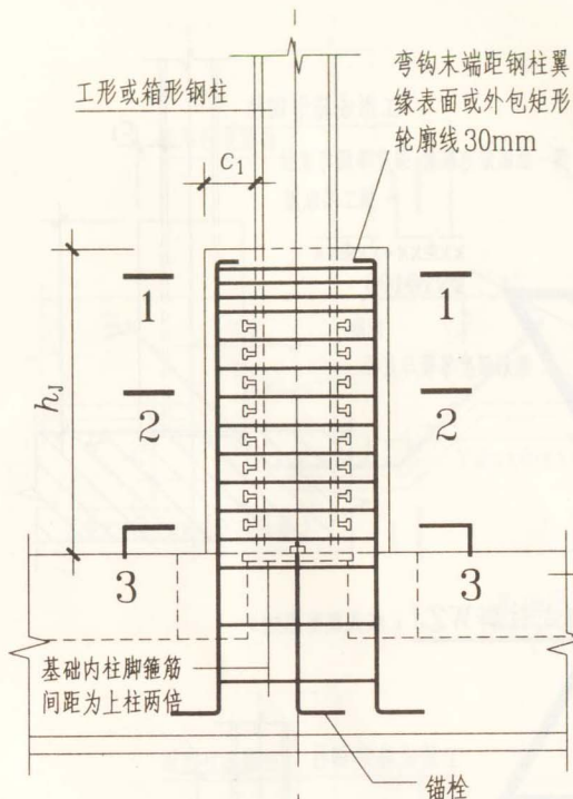
钢柱外包式柱脚WZJ构造 (梁板式筏形基础)
