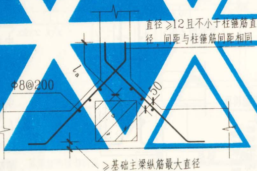
基础主梁偏心穿柱与柱结合部侧腋构造
