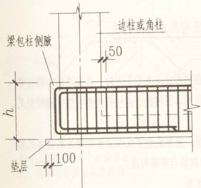
端部无外伸构造(一)
