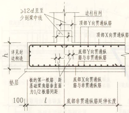
端部等截面外伸构造
