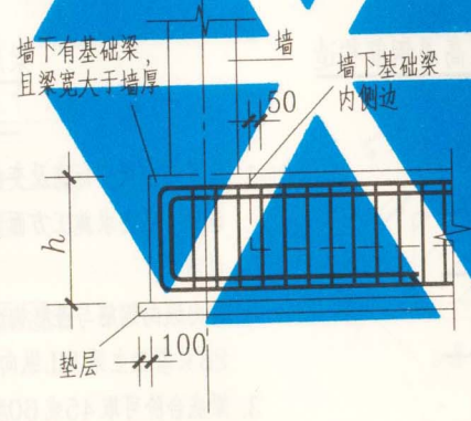
端部无外伸构造(二)
