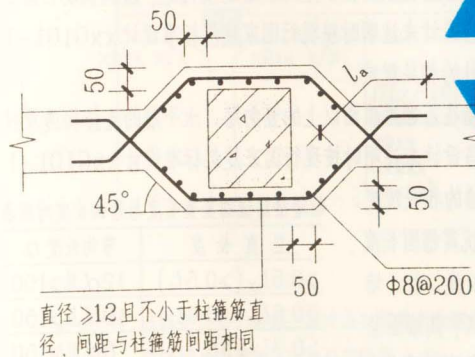
基础主梁中心穿柱侧腋构造
