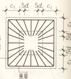
(正方形截面)
