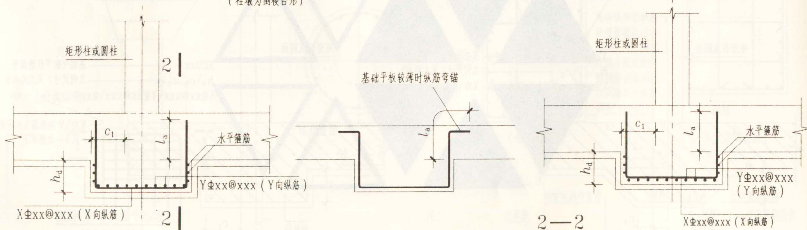
基础平板下柱墩XZD
