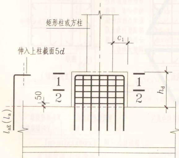
棱柱状上柱墩 SZD
