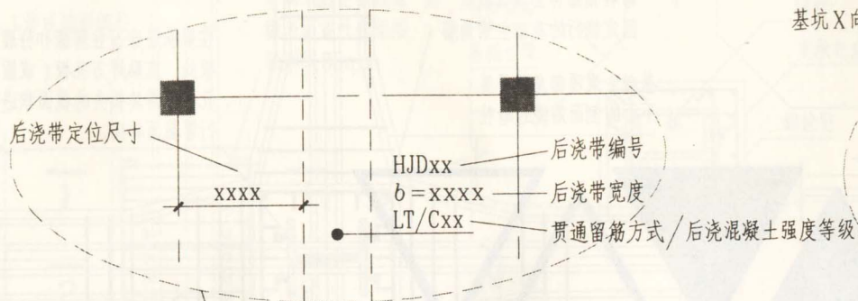
后浇带HJD直接引注
