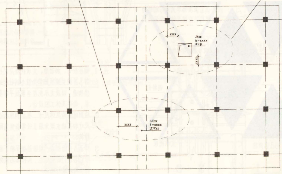
后浇带HJD直接引注
