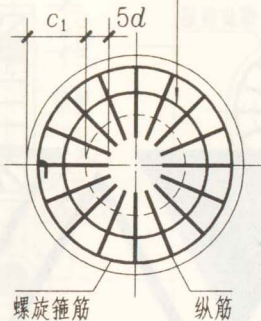
3—3
