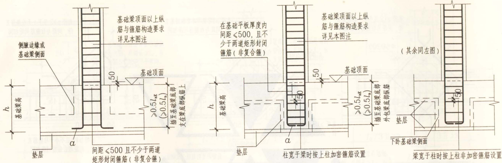
柱插筋构造 (二) (基础梁顶与基础板顶一平)
