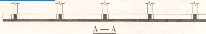
梁板式筏形基础平板LPB标注图示
