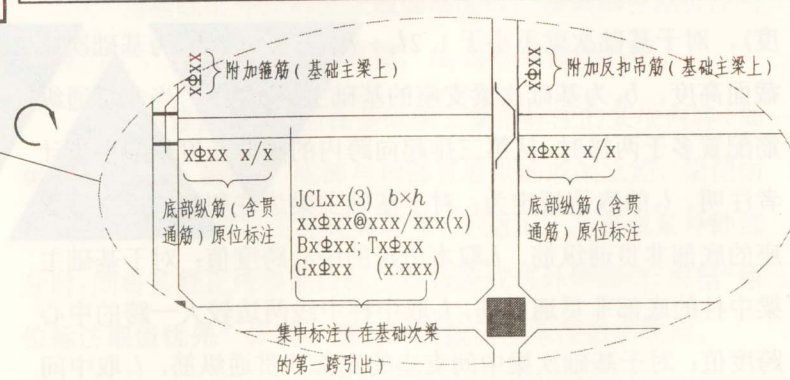
基础主梁JZL与基础次梁JCL标注图示
