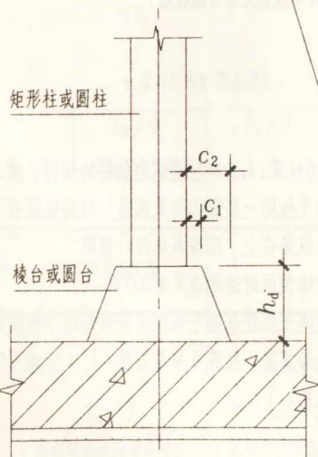
基础平板上柱墩SZD (柱墩为棱台或圆台形状)
