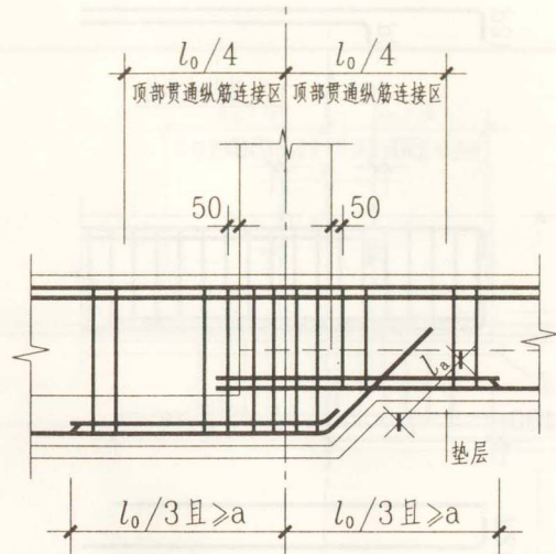
底部第二排筋伸至末端钢筋内侧, 总锚长 \geq l_a ; 当直锚 \geq l_a 时, 可不弯钩。
