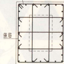
(矩形截面)
