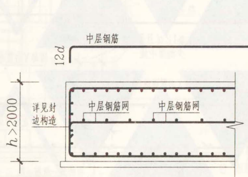
中层筋端头构造
