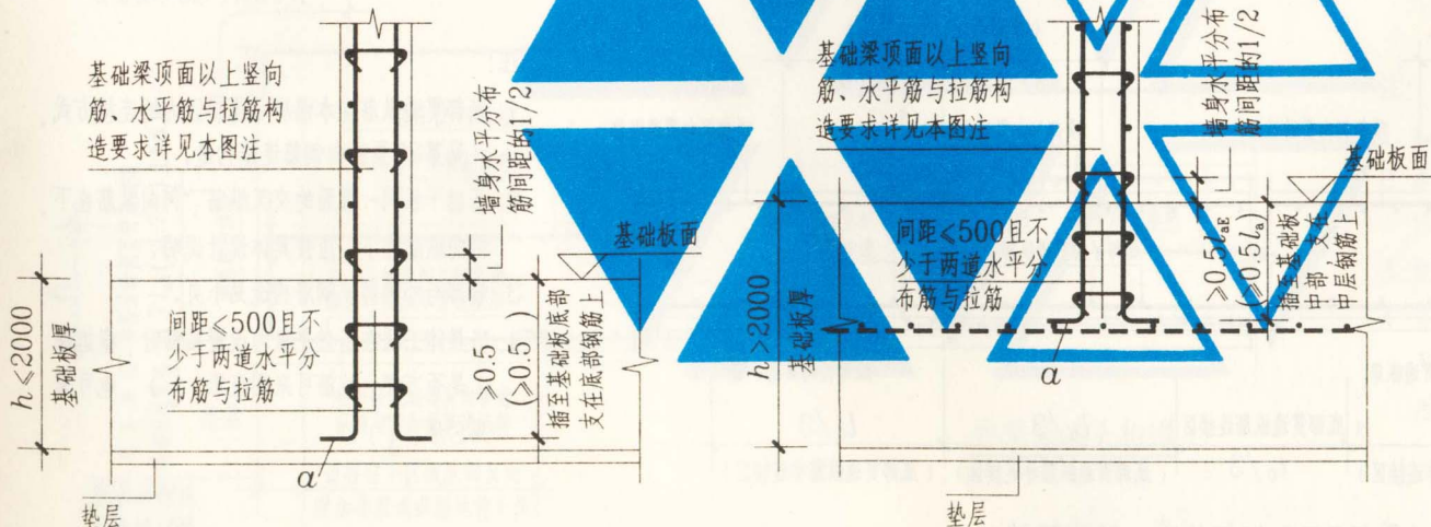
墙插筋构造 (一)
