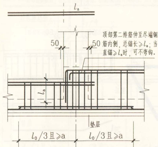
梁顶有高差钢筋构造
