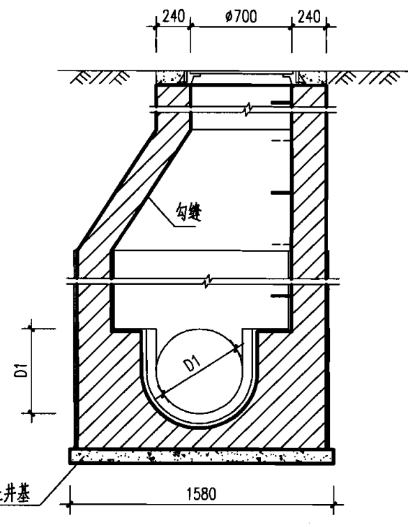
2-2 剖面
