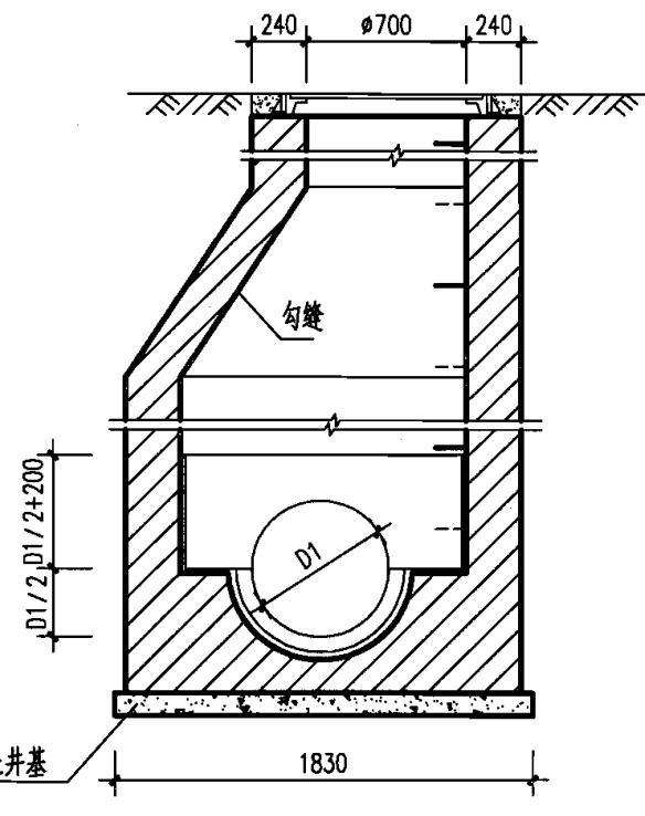
2-2 剖面
