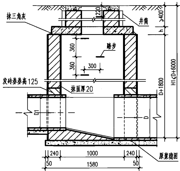
1-1 剖面
