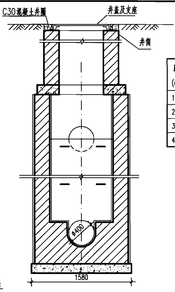
2-2 剖面
