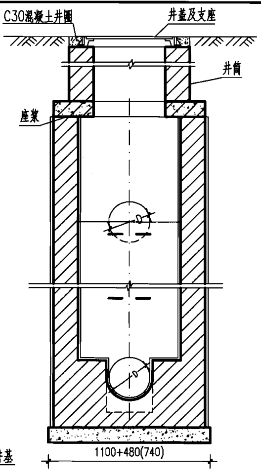
2-2 剖面
