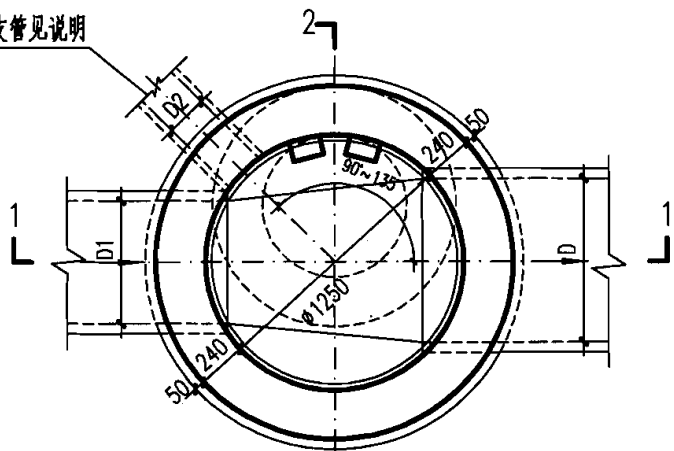
2-1 平面图
