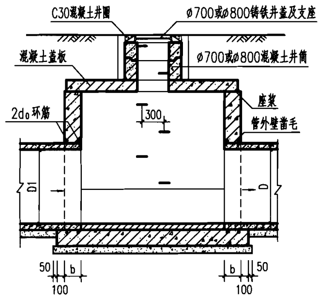
1-1 剖面
