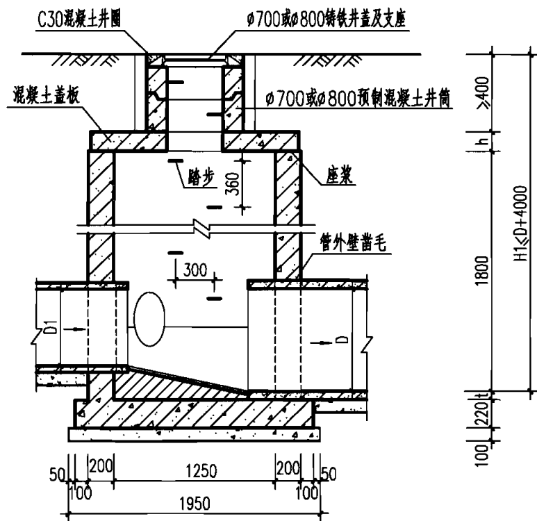
1-1 剖面
