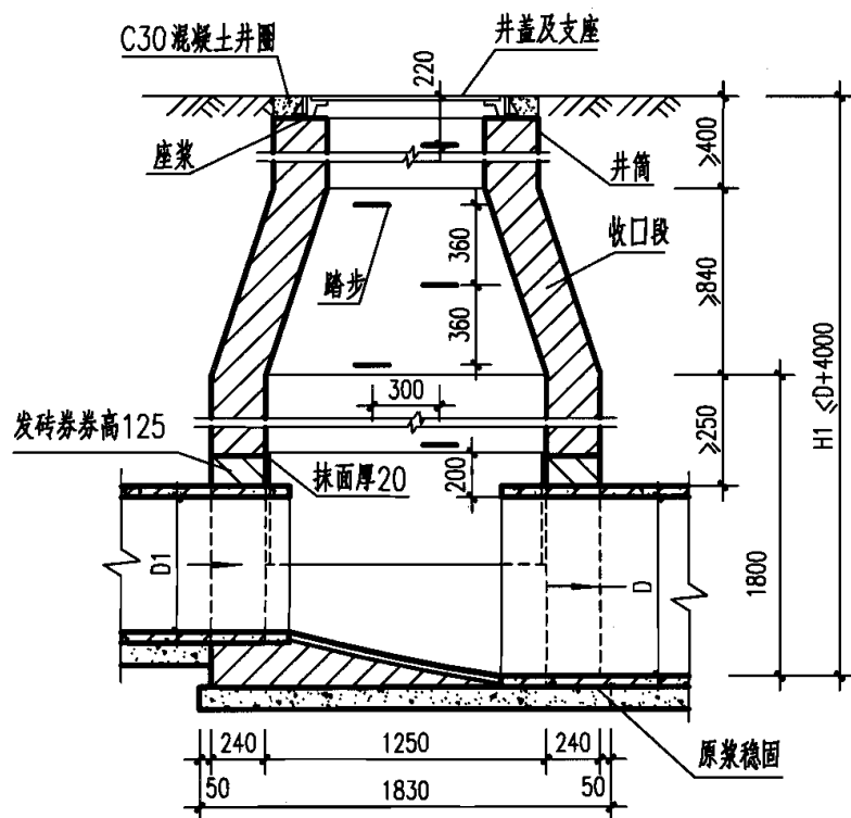
1-1 剖面
