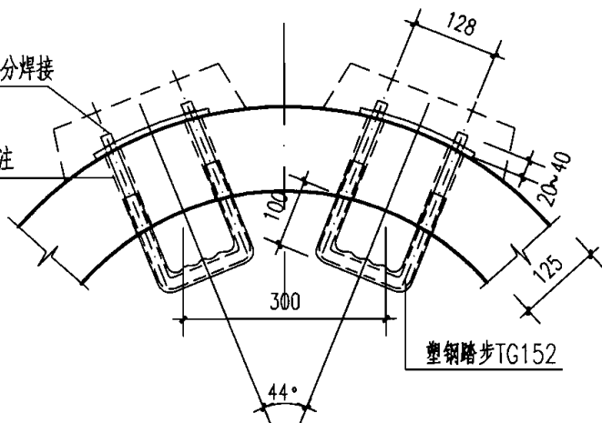
塑钢踏步安装大样
