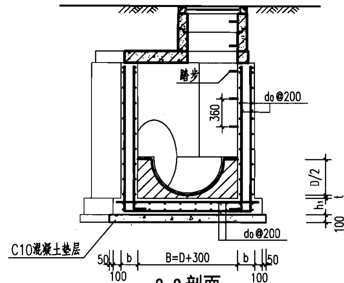
2-2 剖面
