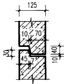
企口尺寸大样
