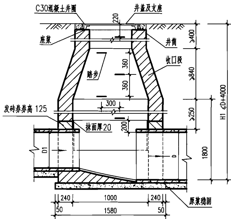
1-1 剖面
