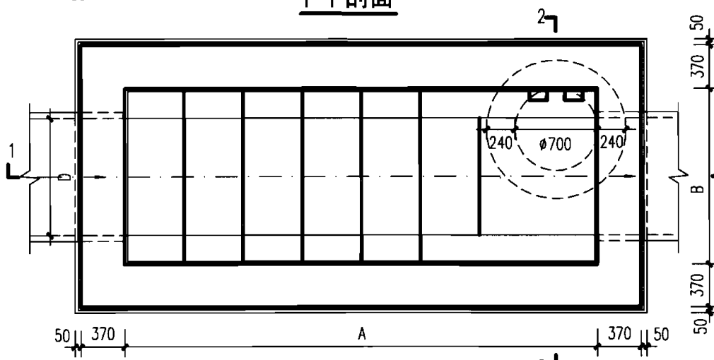
平面图
