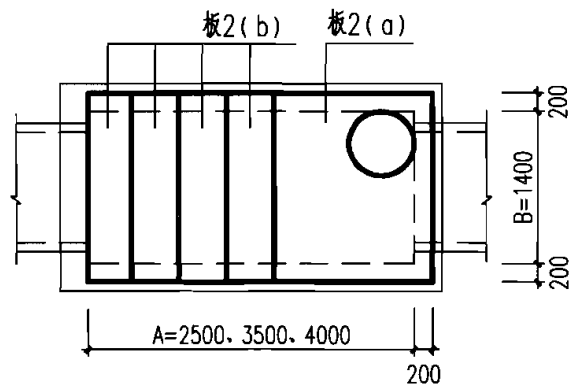
盖板布置图
