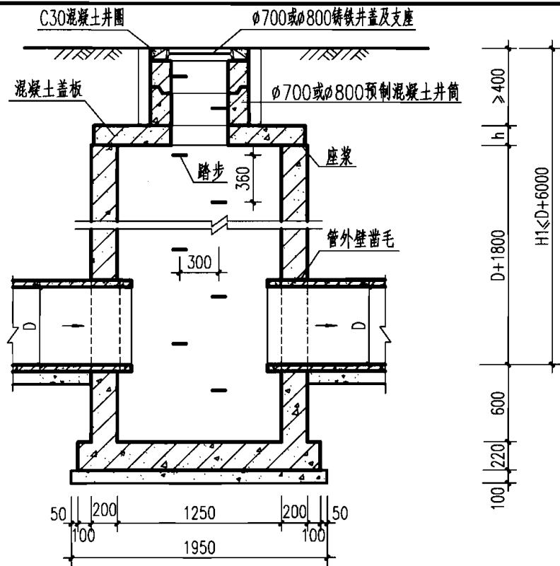
1-1 剖面
