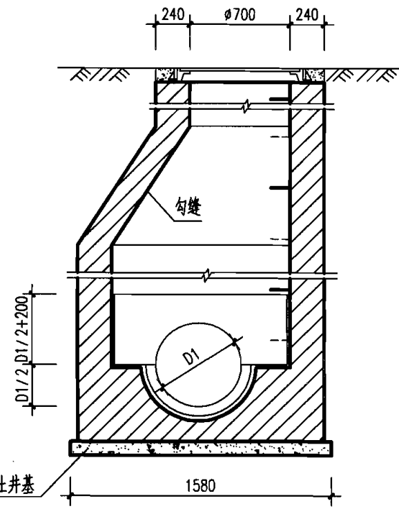
2-2 剖面
