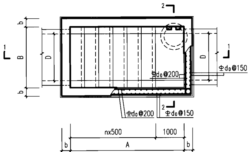
井室平面图 1:50
