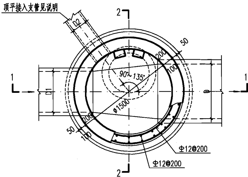
平面图
