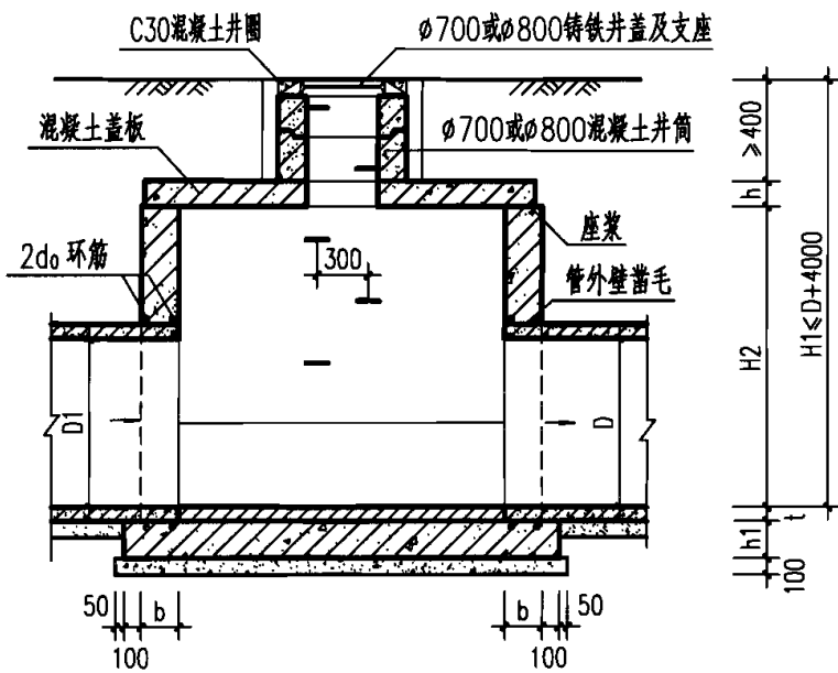
1-1 剖面
