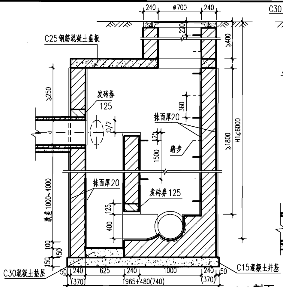
1-1 剖面
