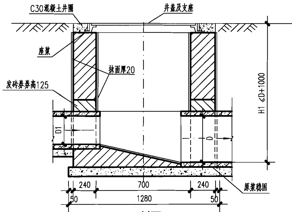
1-1 剖面
