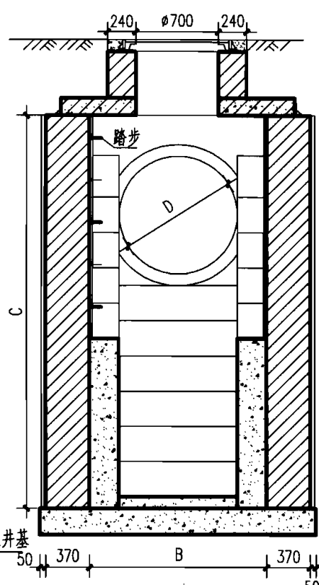
2-2 剖面
