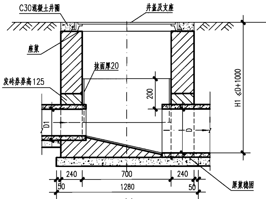
1-1 剖面
