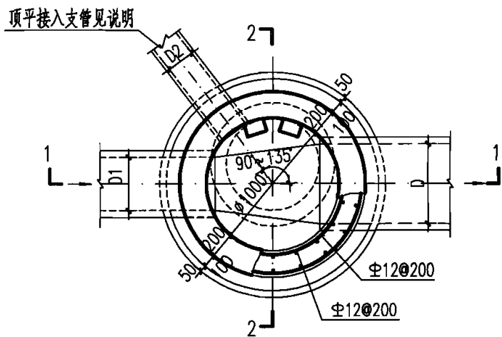
平面图
