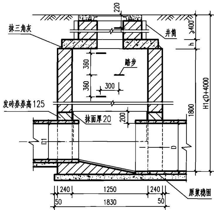
1-1 剖面
