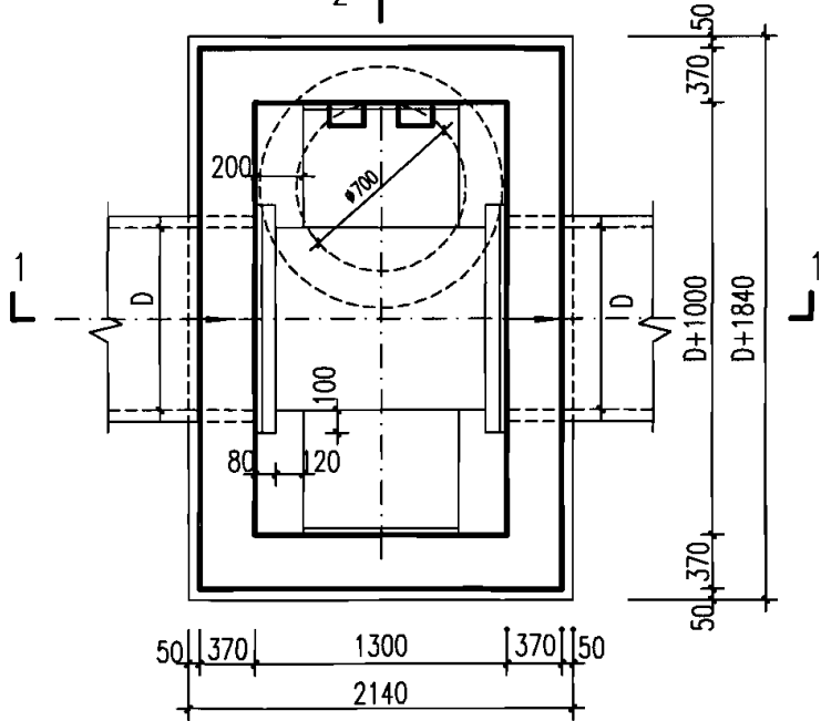
2 平面图
