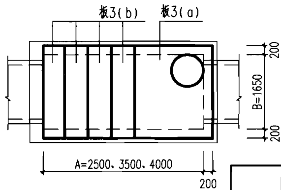
盖板布置图
