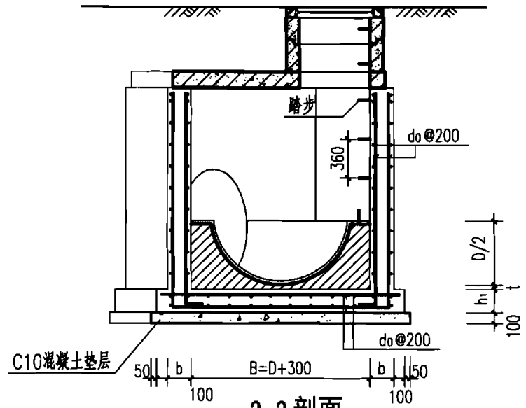
2-2 剖面
