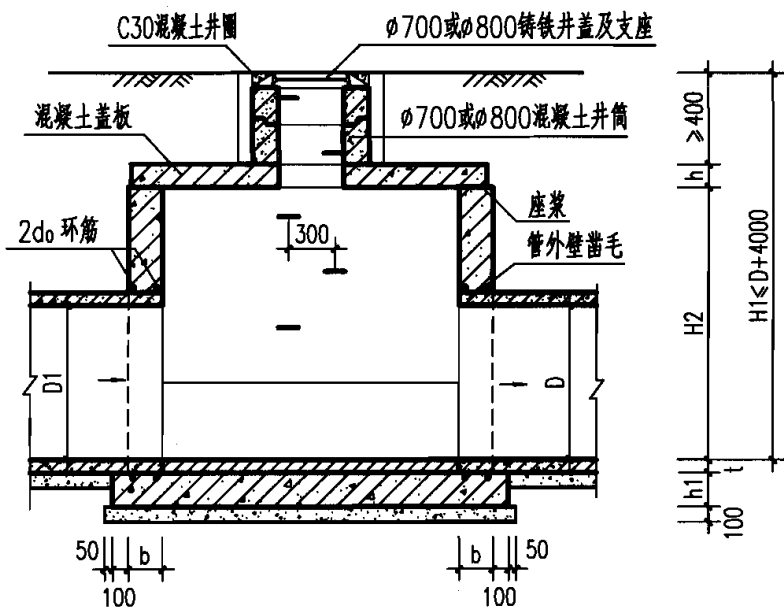
1-1 剖面
