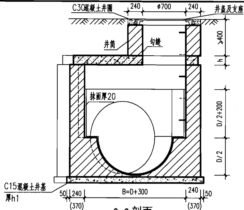
2-2 剖面
