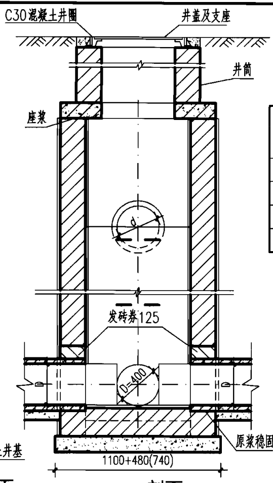
2-2 剖面
