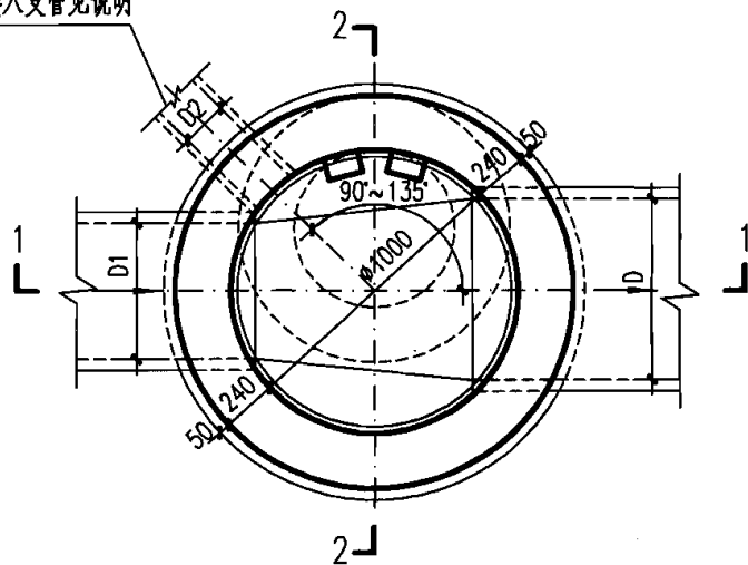
平面图
