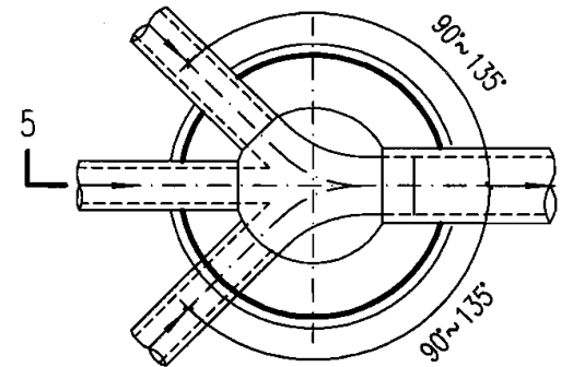
90° ~ 135°四通井平面图
