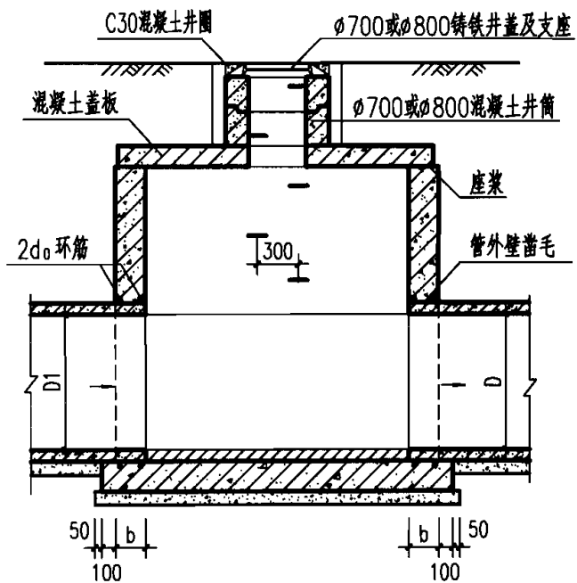
1-1 剖面
