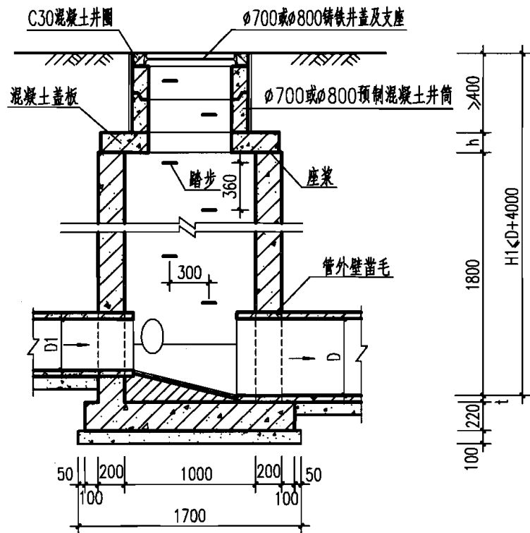
1-1 剖面
