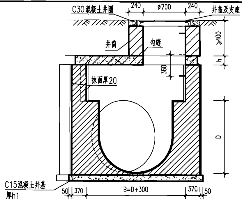
2-2 剖面
