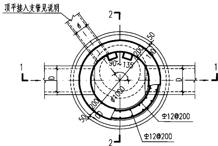
平面图
