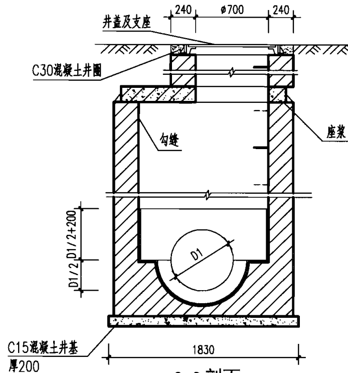
2-2 剖面
