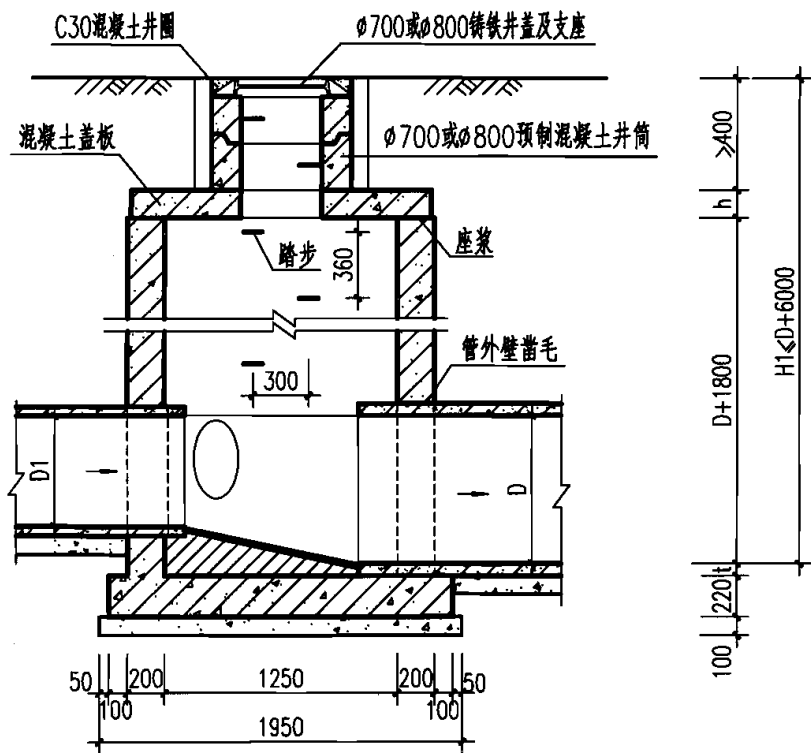
1-1 剖面
