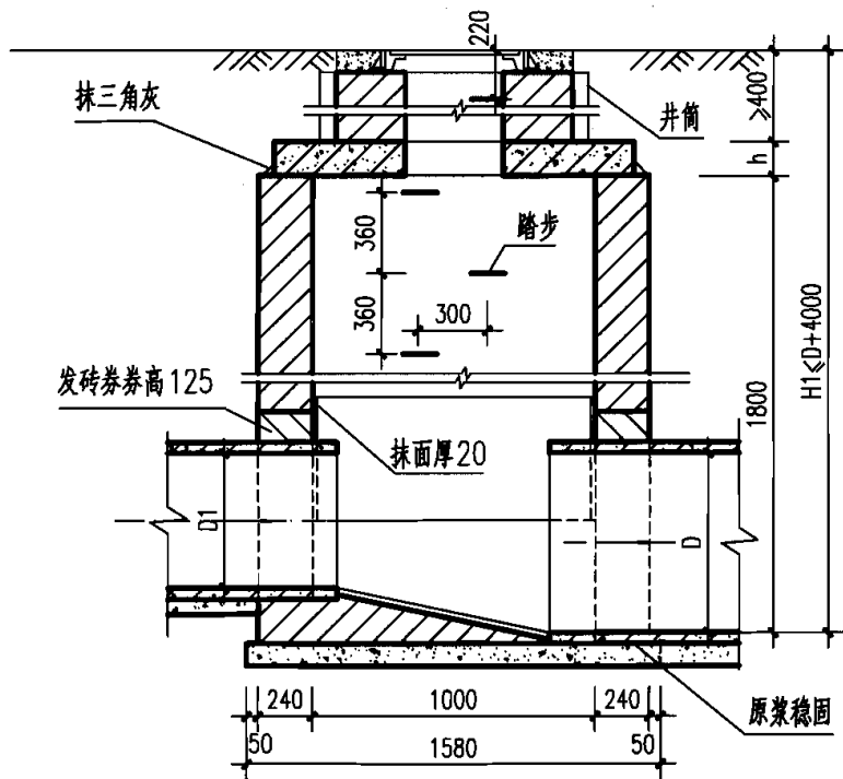
1-1 剖面
