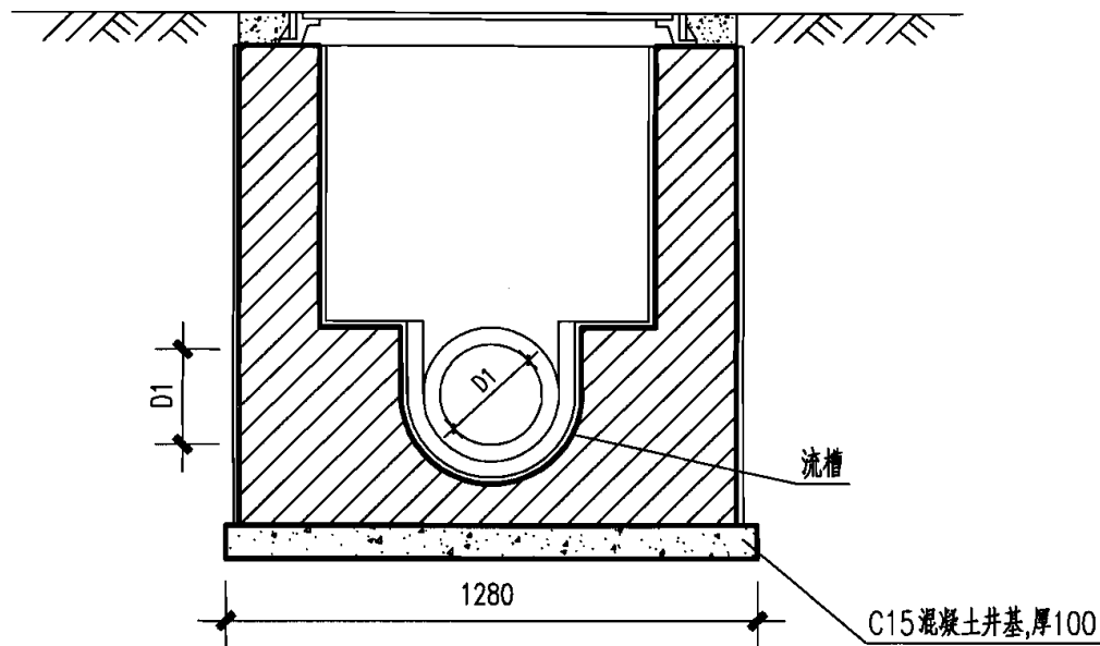
2-2 剖面
