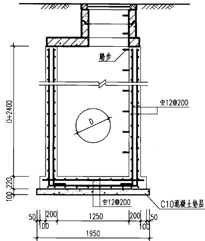
2-2 剖面
