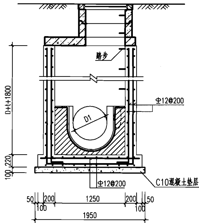
2-2 剖面
