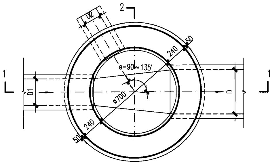
平面图
