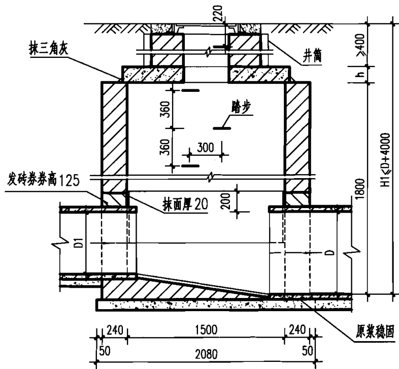
1-1 剖面
