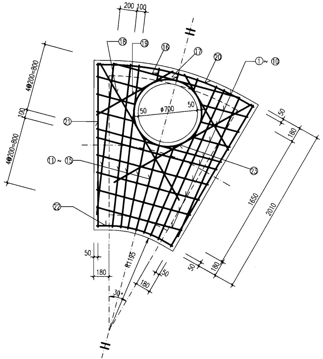
扇形雨污水检查井 (150°) 盖板配筋图 ③ ( D=1200 \sim 1350 )
