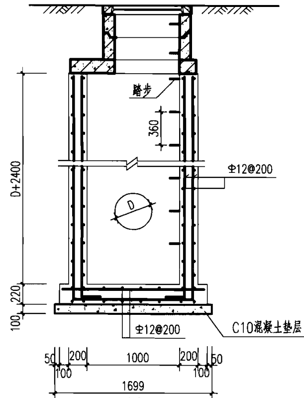
2-2 剖面
