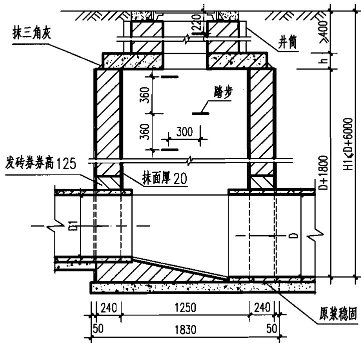
1-1 剖面
