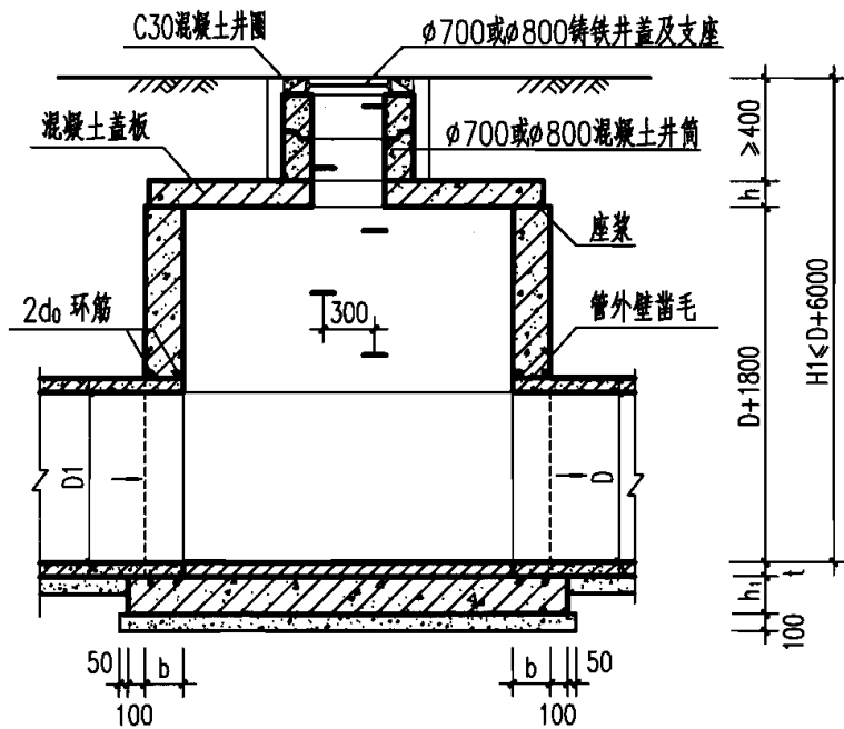
1-1 剖面
