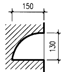
1-1剖面
