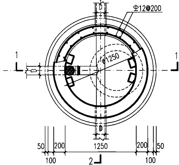
2-2 剖面
