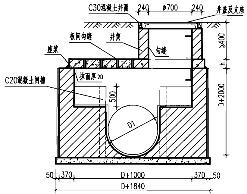
2-2 剖面
