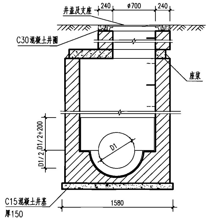
2-2 剖面
