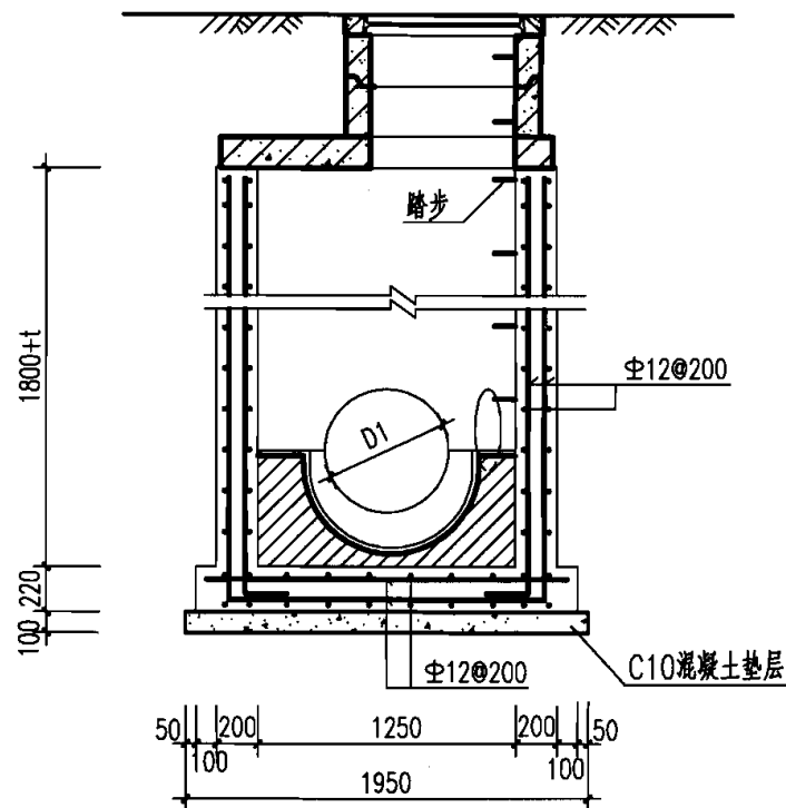
2-2 剖面
