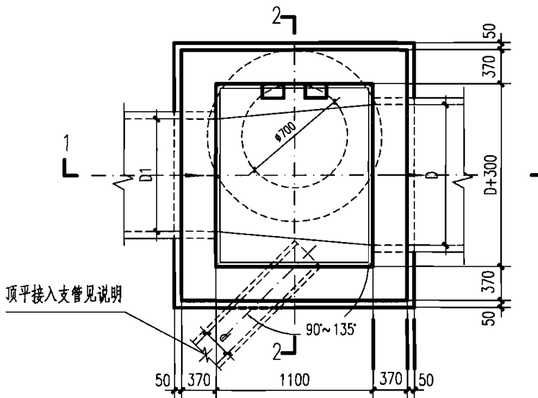
平面图
