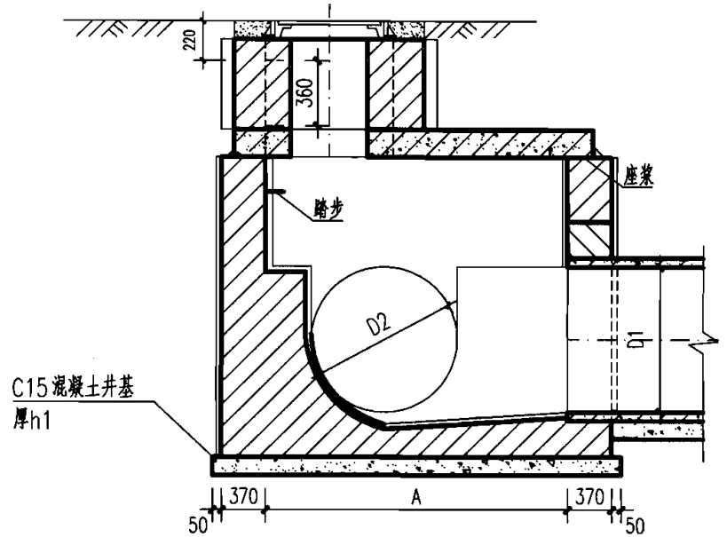
2-2 剖面
