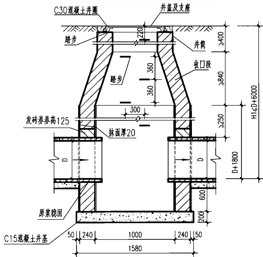
1-1 剖面
