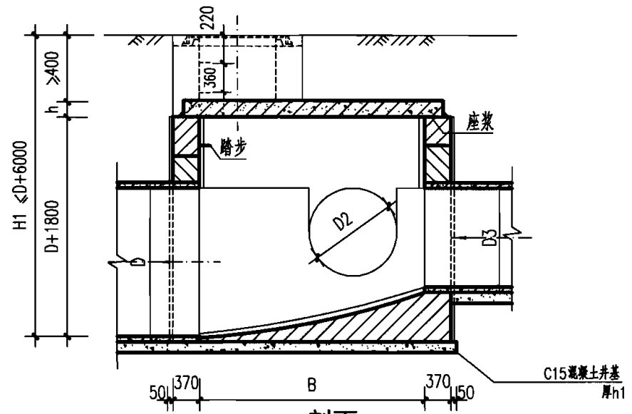
2-2 剖面
