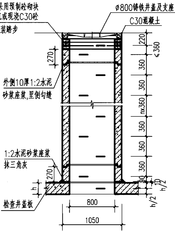
预制井筒安装大样
