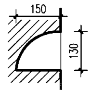
1-1剖面
