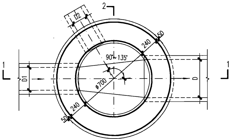
2 平面图
