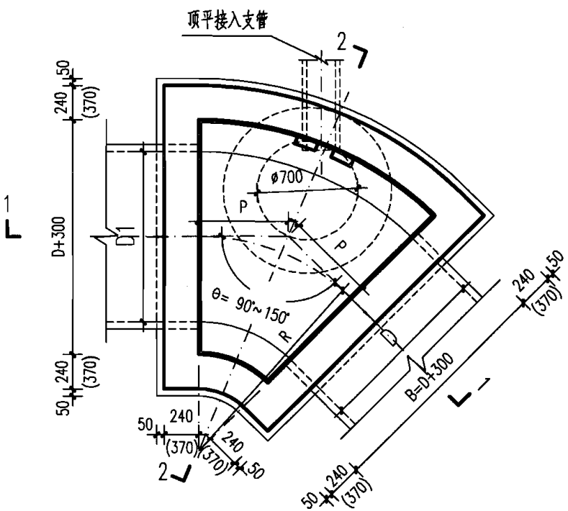
平面图
