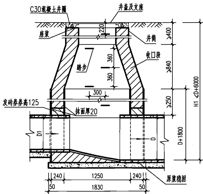
1-1 剖面
