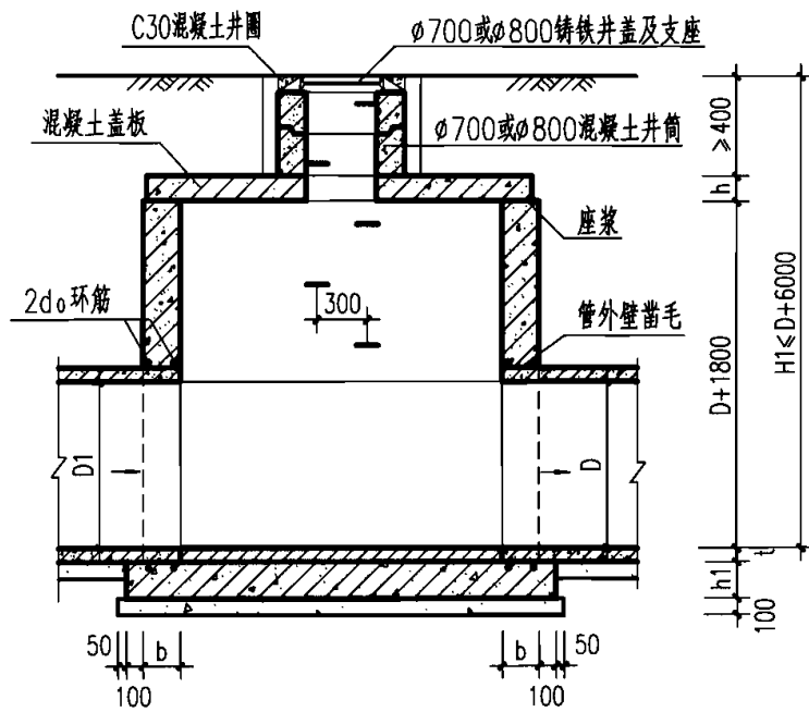
1-1 剖面
