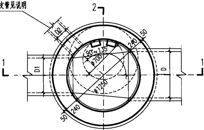
2 平面图
