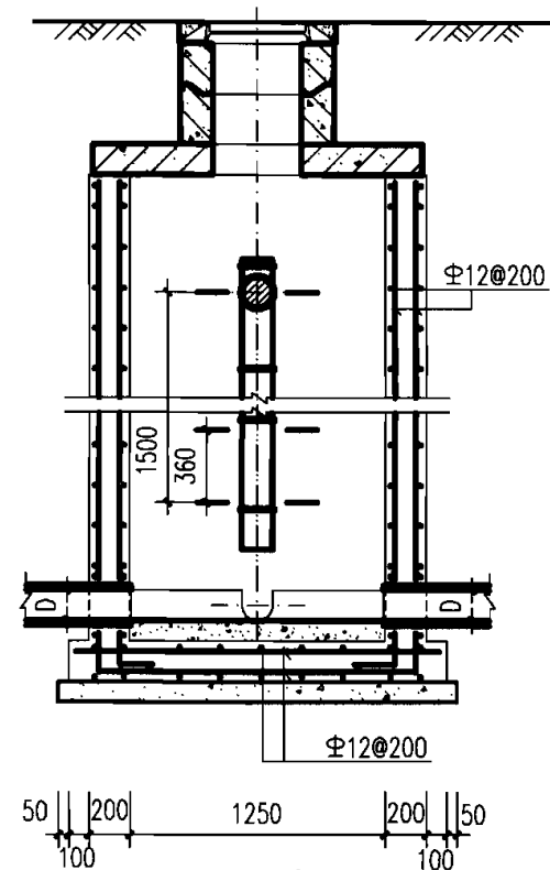
2-2 剖面
