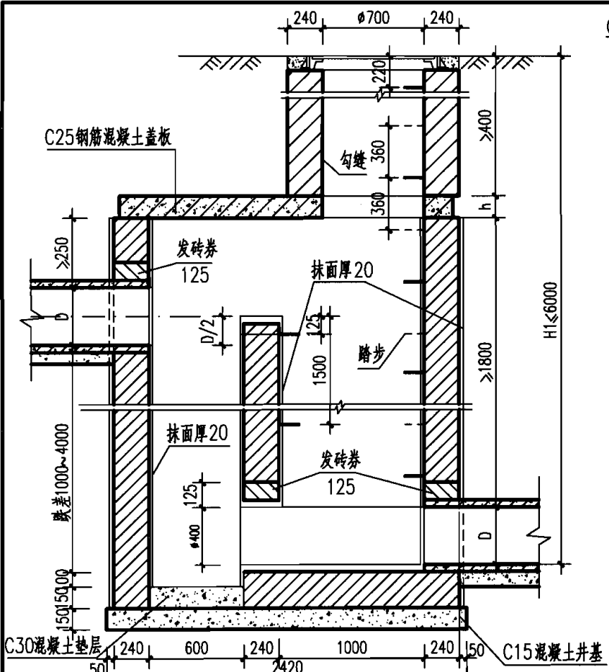
1-1 剖面
