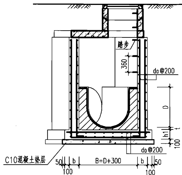
2-2 剖面
