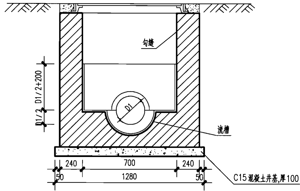
2-2 剖面
