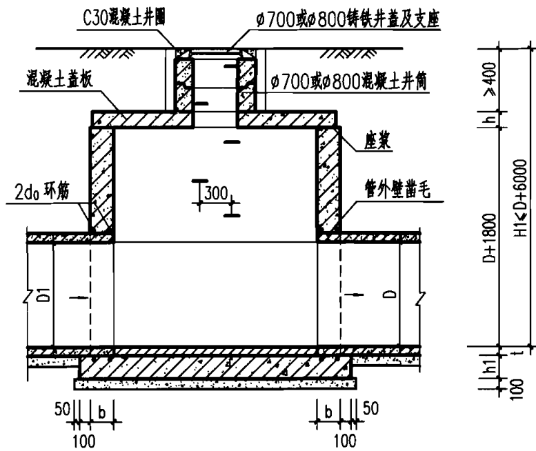
1-1 剖面
