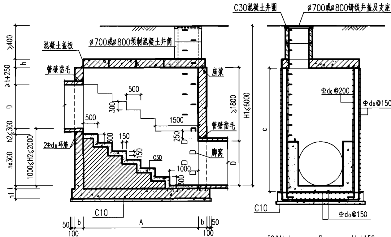
1-1 剖面 1:50
