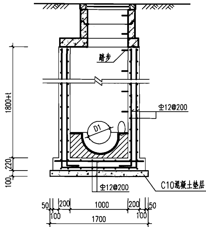
2-2 剖面
