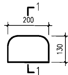
脚窝立面
