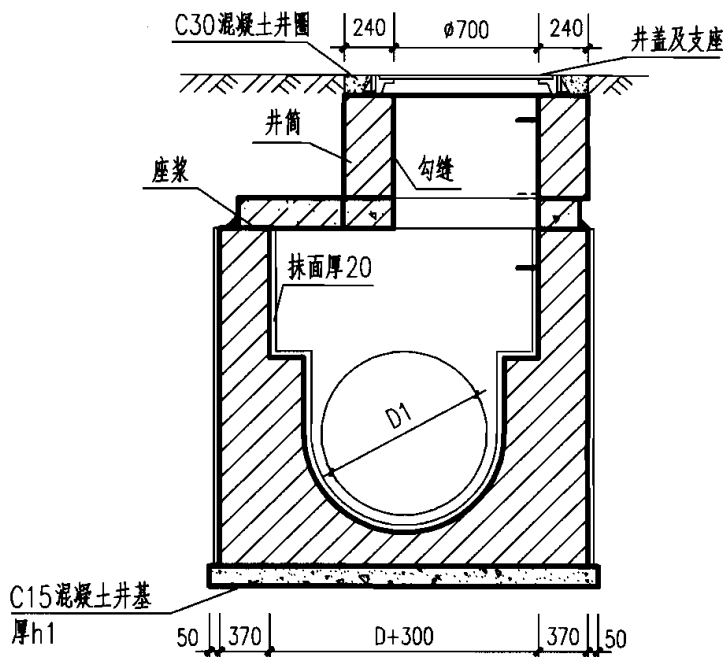
2-2 剖面
