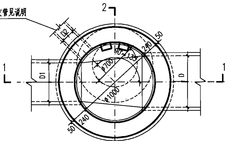
2-1 平面图
