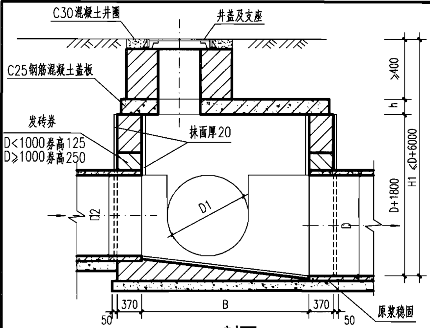
1-1 剖面
