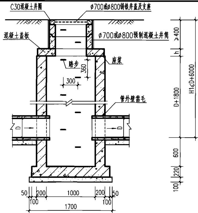
1-1 剖面
