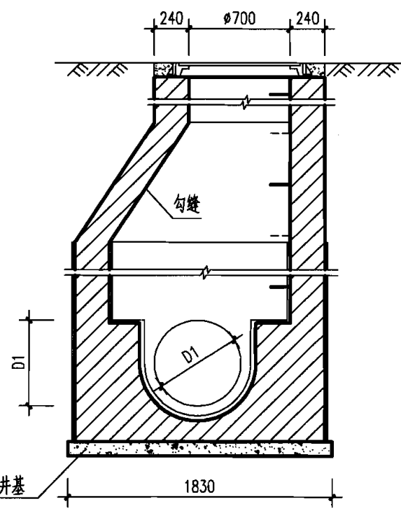
2-2 剖面
