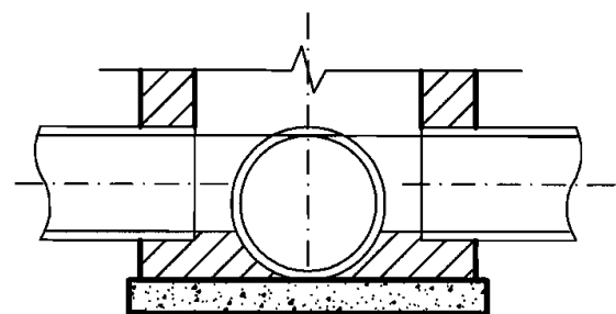
3-3
