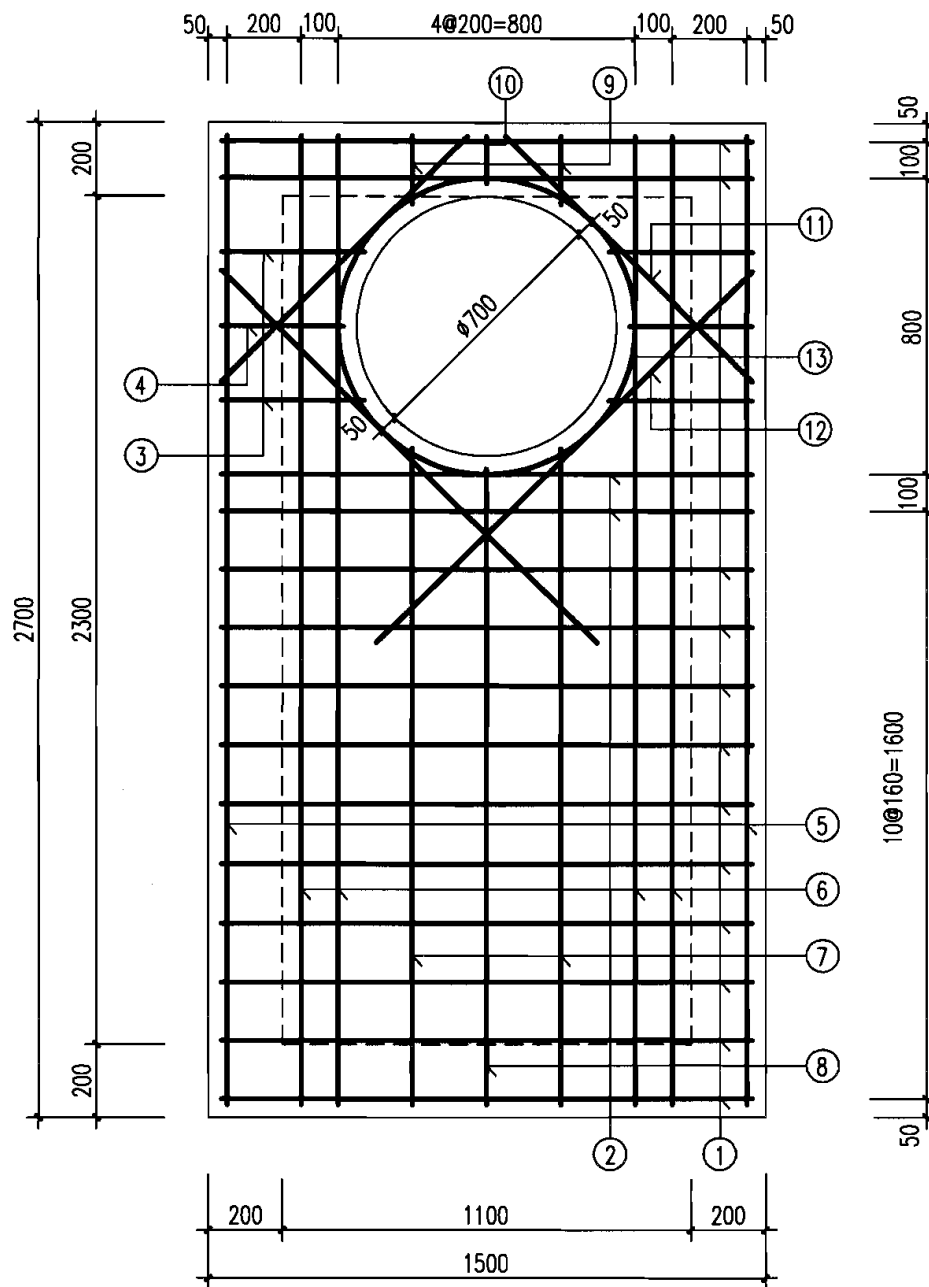
矩形直线雨污水检查井盖板配筋图 ⑤ (D=2000)
