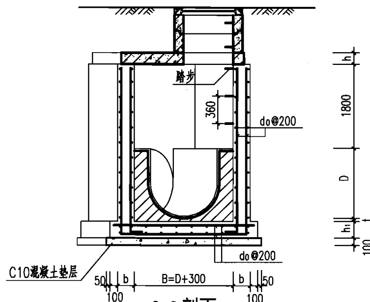
2-2 剖面
