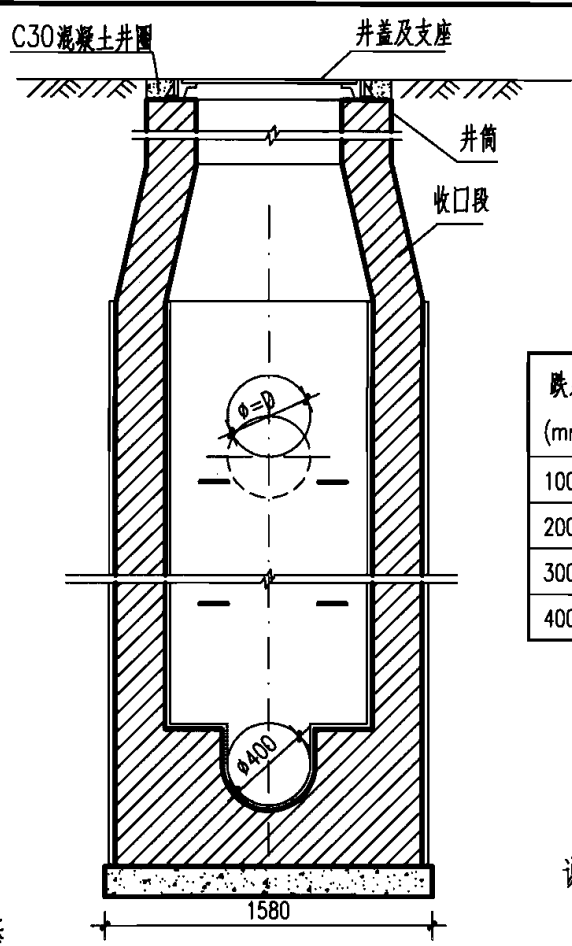
2-2 剖面
