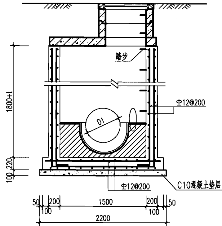
2-2 剖面
