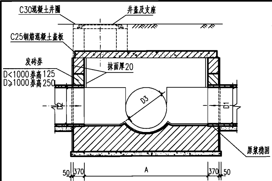
1-1 剖面
