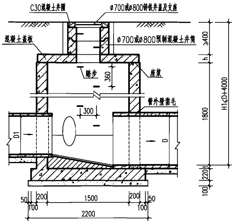
1-1 剖面
