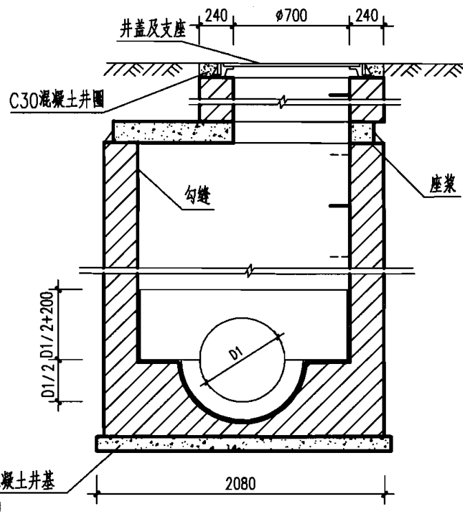
2-2 剖面
