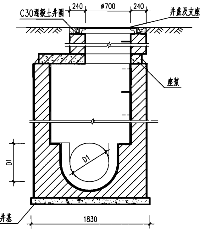
2-2 剖面
