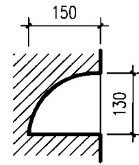
1-1剖面
