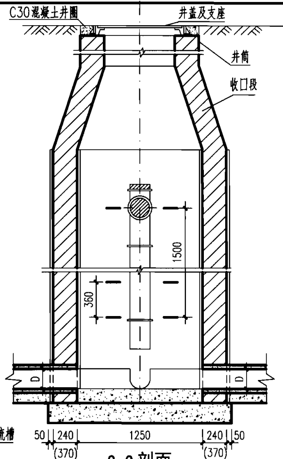
2-2 剖面
