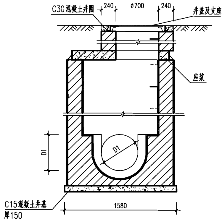
2-2 剖面
