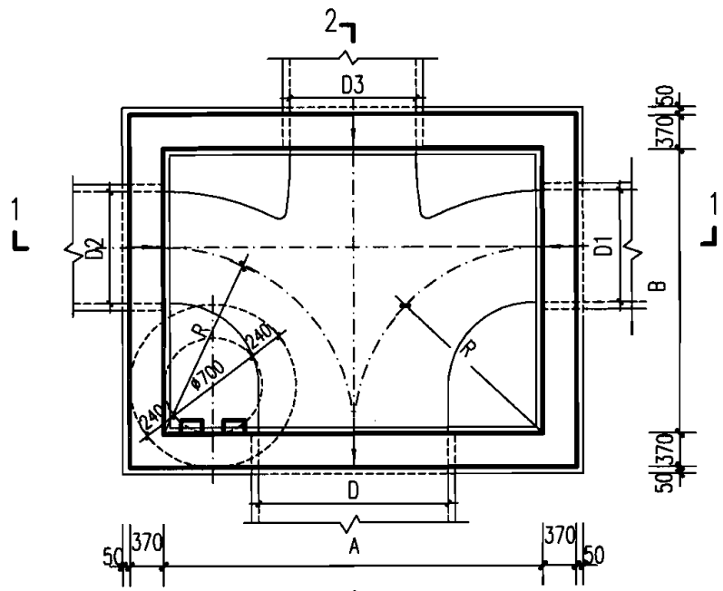
平面图
