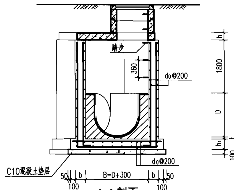
2-2 剖面
