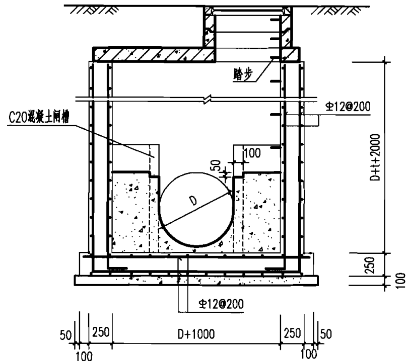
2-2 剖面
