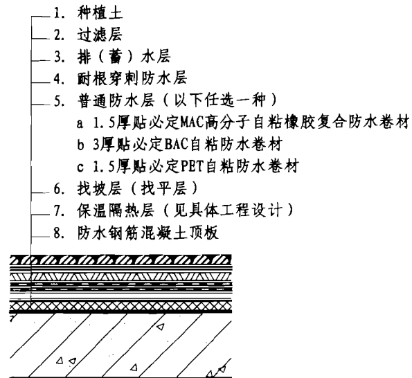
③ 地下室种植顶板防水构造（一级设防）
