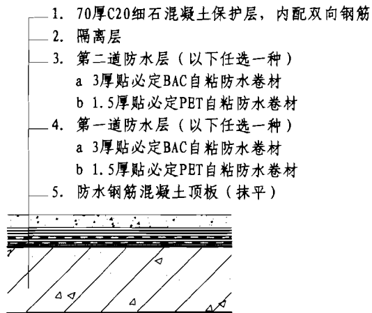
①地下室顶板一级防水构造
