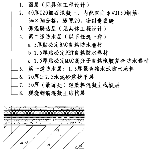
② 倒置式平屋面I级防水构造
