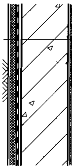
① 地下室外墙一级防水构造（外防外贴）
