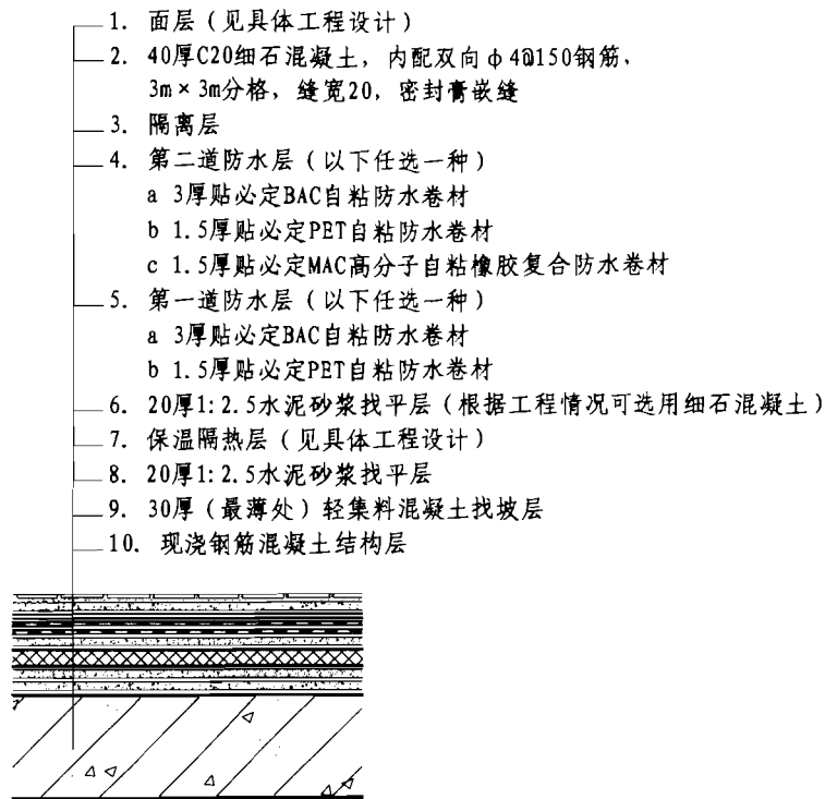
① 正置式平屋面I级防水构造
