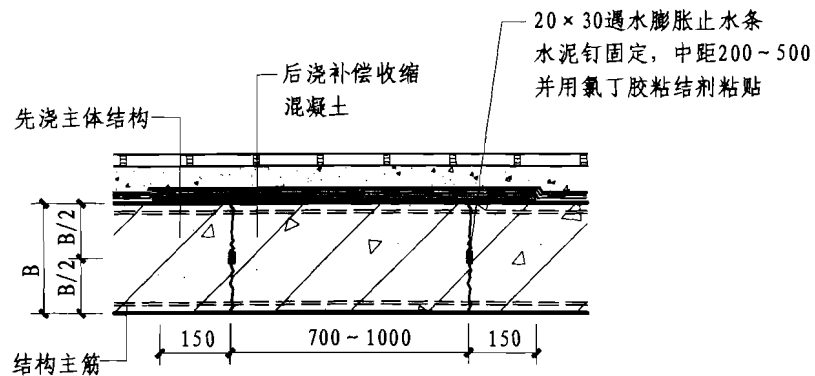
② 顶板后浇带
