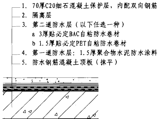
③地下室顶板一级防水构造
