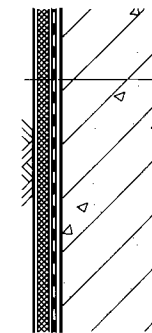
④ 地下室外墙二级防水构造（外防外涂）
