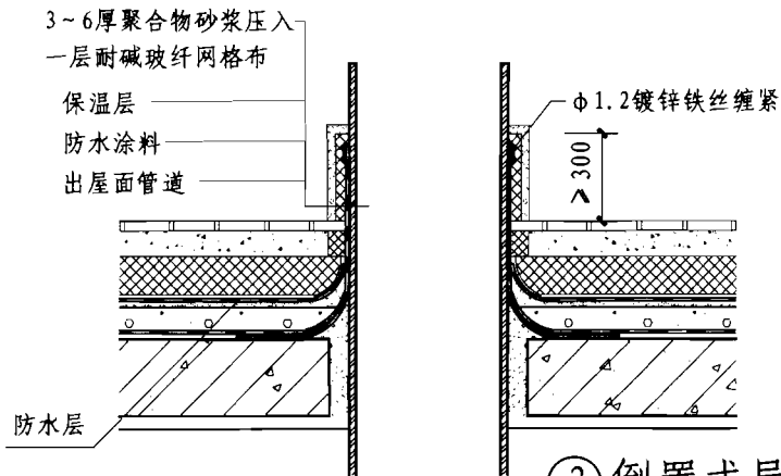
② 倒置式屋面出屋面管道
