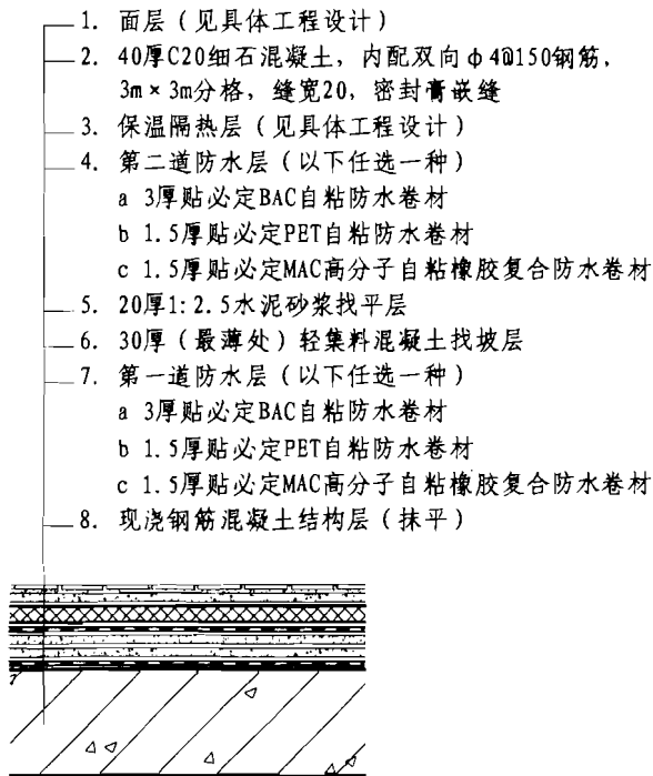
① 倒置式平屋面I级防水构造
