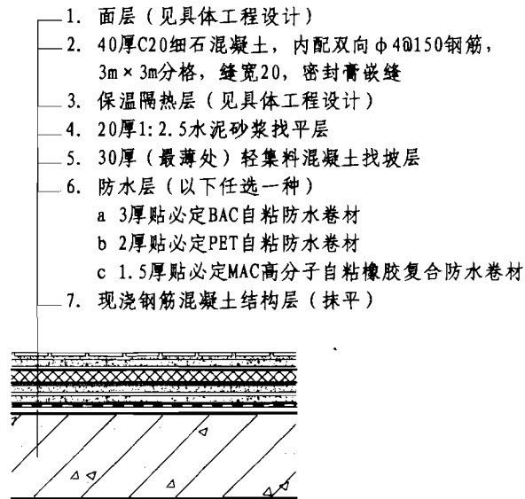
② 倒置式平屋面II级防水构造
