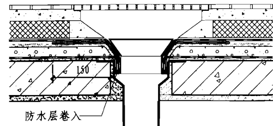
③ 倒置式屋面直式水落口
