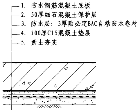
①地下室底板二级防水构造
