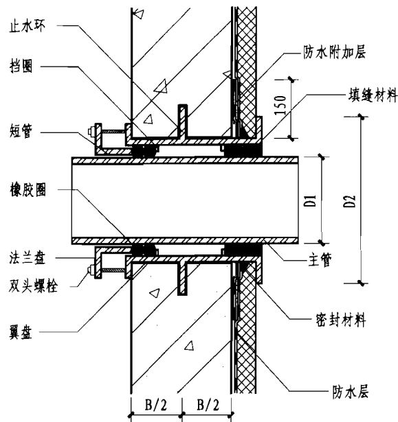
③ 套管式穿墙管
