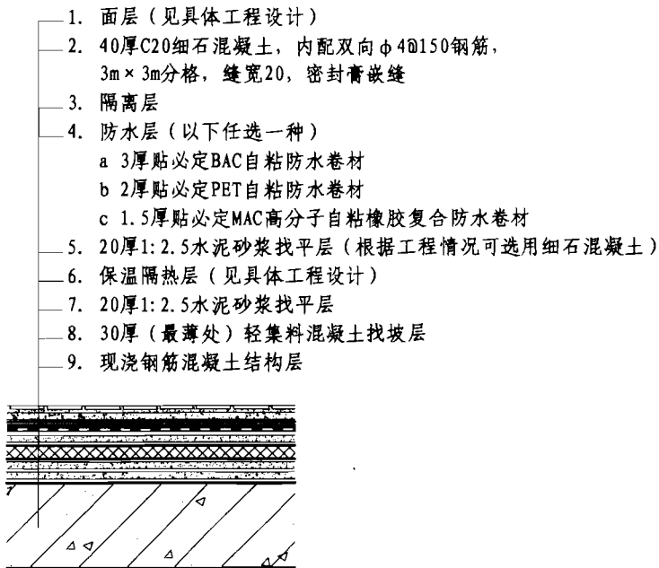
① 正置式平屋面II级防水构造
