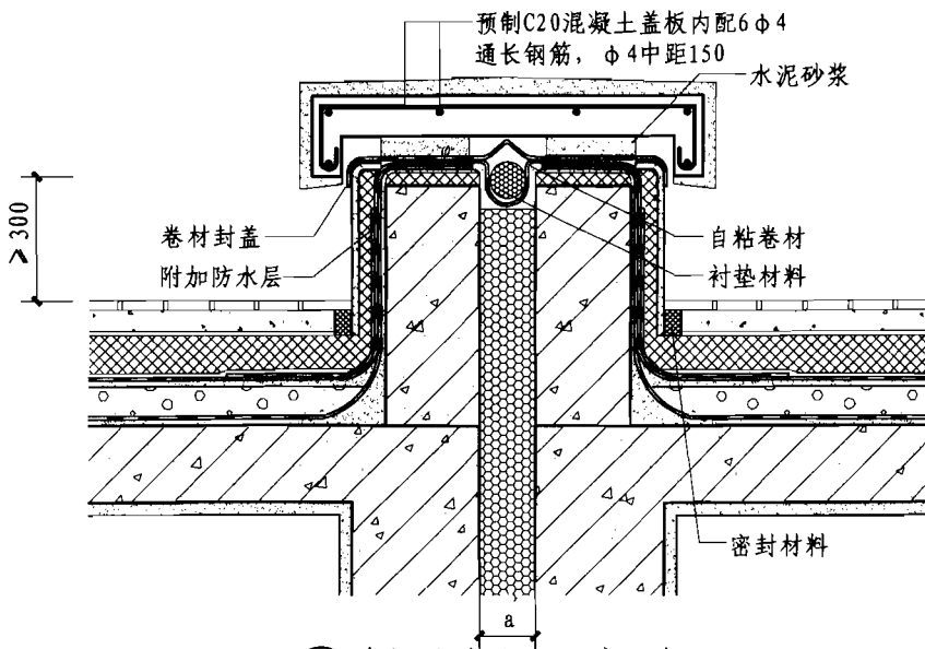
② 倒置式屋面出屋面管道
